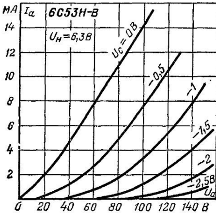
Анодные характеристики.
