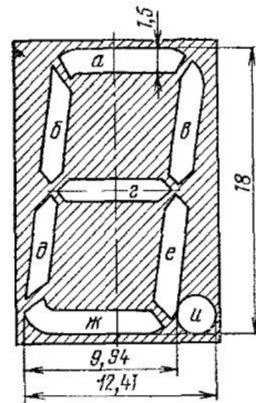
Расположение и условное обозначение анодов-сегментов ИБ-22
